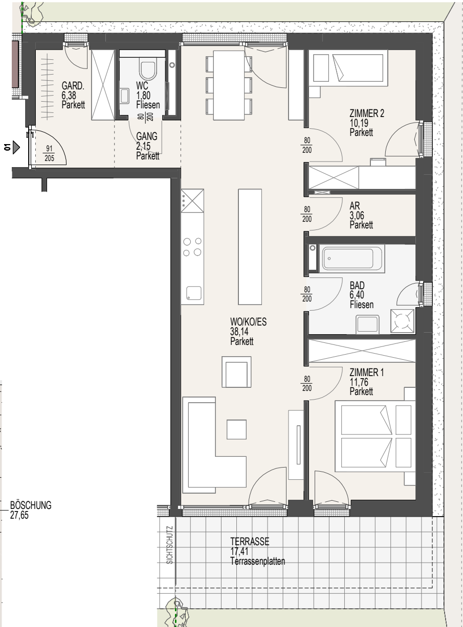
TOP 01 | 1 : 100
